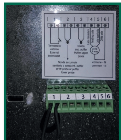
Anschlüsse für externe Fühler und Thermostat
